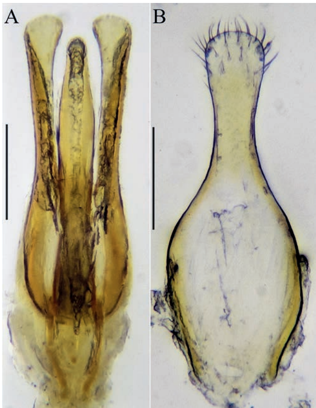
Fig. 6 – Male Anthrenus senegalensis . A) Aedeagus dorsal aspect; B) sternite IX. Scale bar = 100 µm in both cases. / Maschio di Anthrenus senegalensis . A) Vista dorsale dell'edeago; B) sternite IX. Scala grafica = 100 µm in entrambi i casi.
